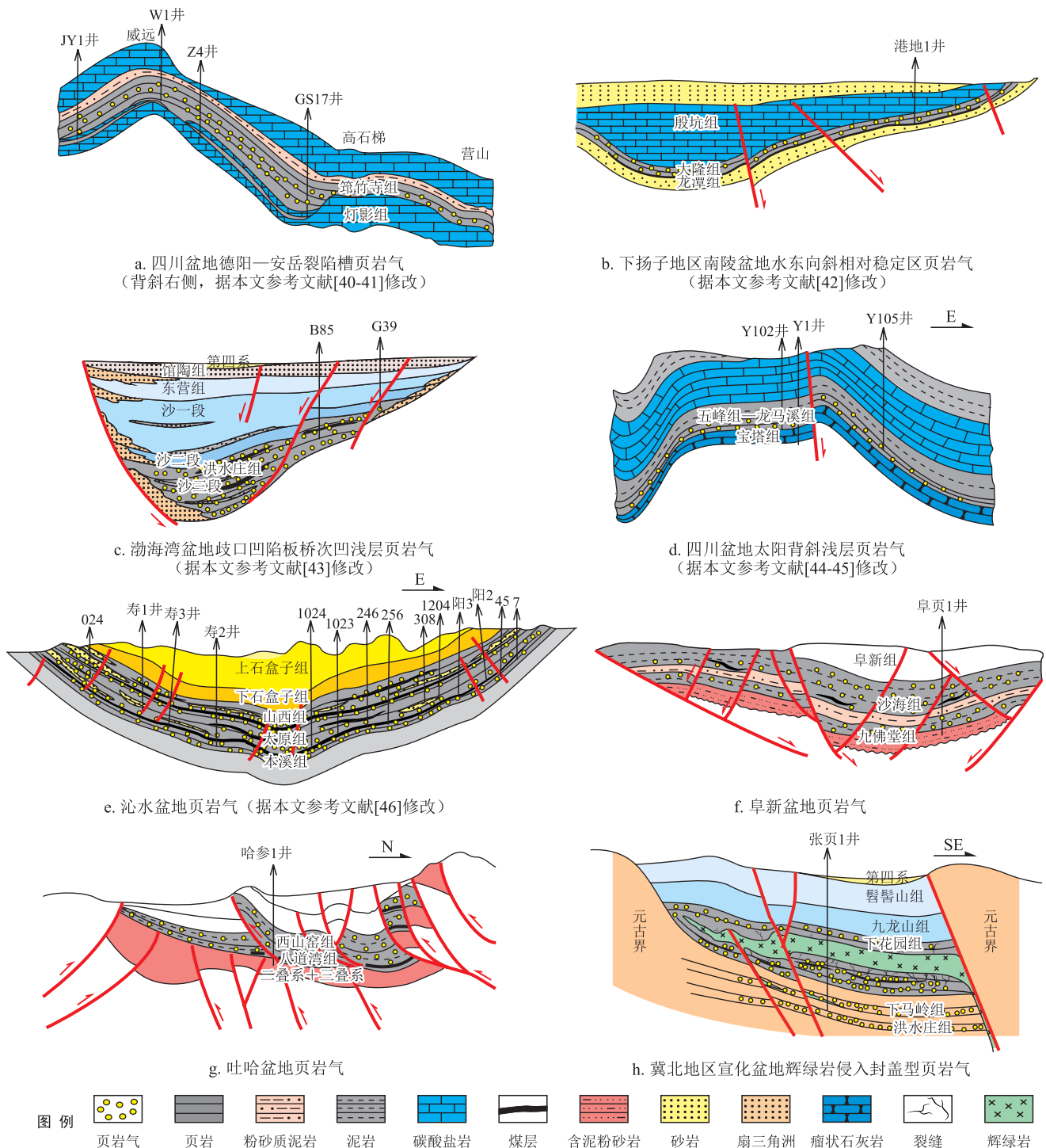
图 1 特殊类型页岩气成藏模式图
